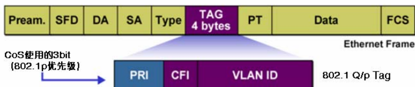
图 9-2 802.1Q的帧格式
